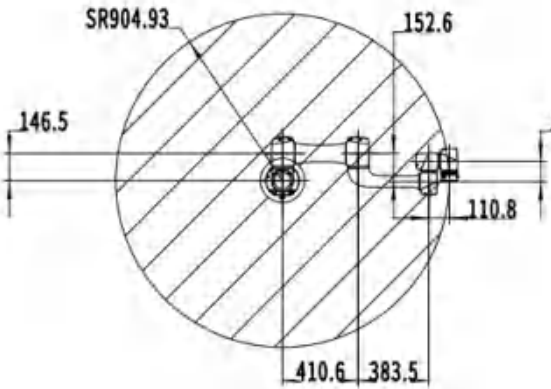
CRP-RC09-05
