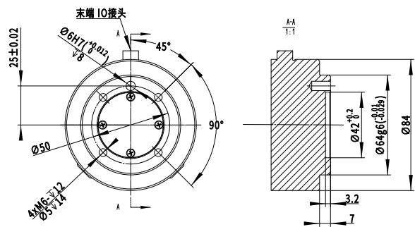
CRP-RC09-05/CRP-RC18-05
